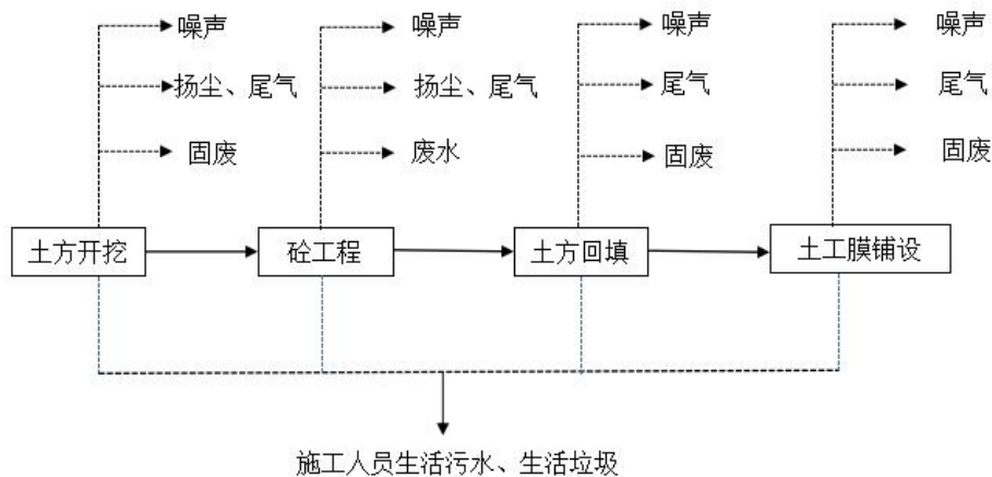
图 4-5 护坡护岸工程施工工艺及产污节点图
