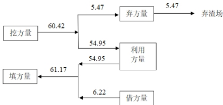
图 4-2 项目土石方平衡图 单位：万 m 3
